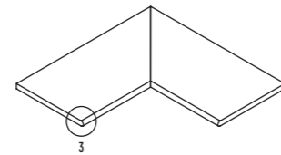
Canto interior boleado Bullnose inner corner Margelle avec bord intérieur arrondi Abgerundete Innenecke (Gärung) 30x60 20MM AS LP-6660 30x60 RET. 20MM AS LP-6660 (vendida ao par . sold per two pieces set . vendue à la paire . Paarweise verkauft)
